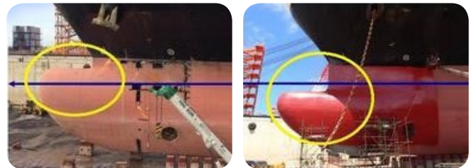
▲ 改造前 ▲ 改造後 バルバスパウの改造（船型や運航条件に併せてバルバスパウの形を改造）
